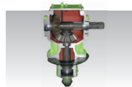
Robustní úhlové převodovky 210 koní
