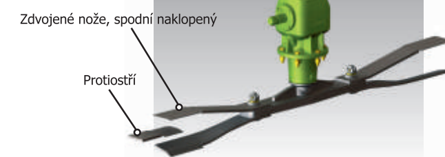
FX - 742 provedení se zdvojenými noži pohled bez pláště
